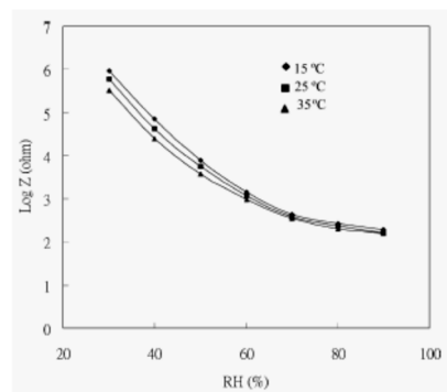
Rys. 5. Zależność impedancji w funkcji wilgotności w różnej temperaturze.
