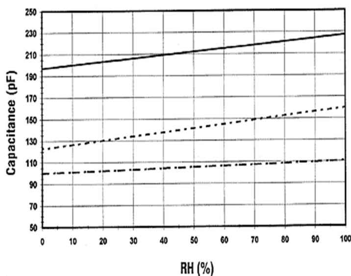
Rys. 2. Przykładowe zmiany pojemności w funkcji wilgotności.
